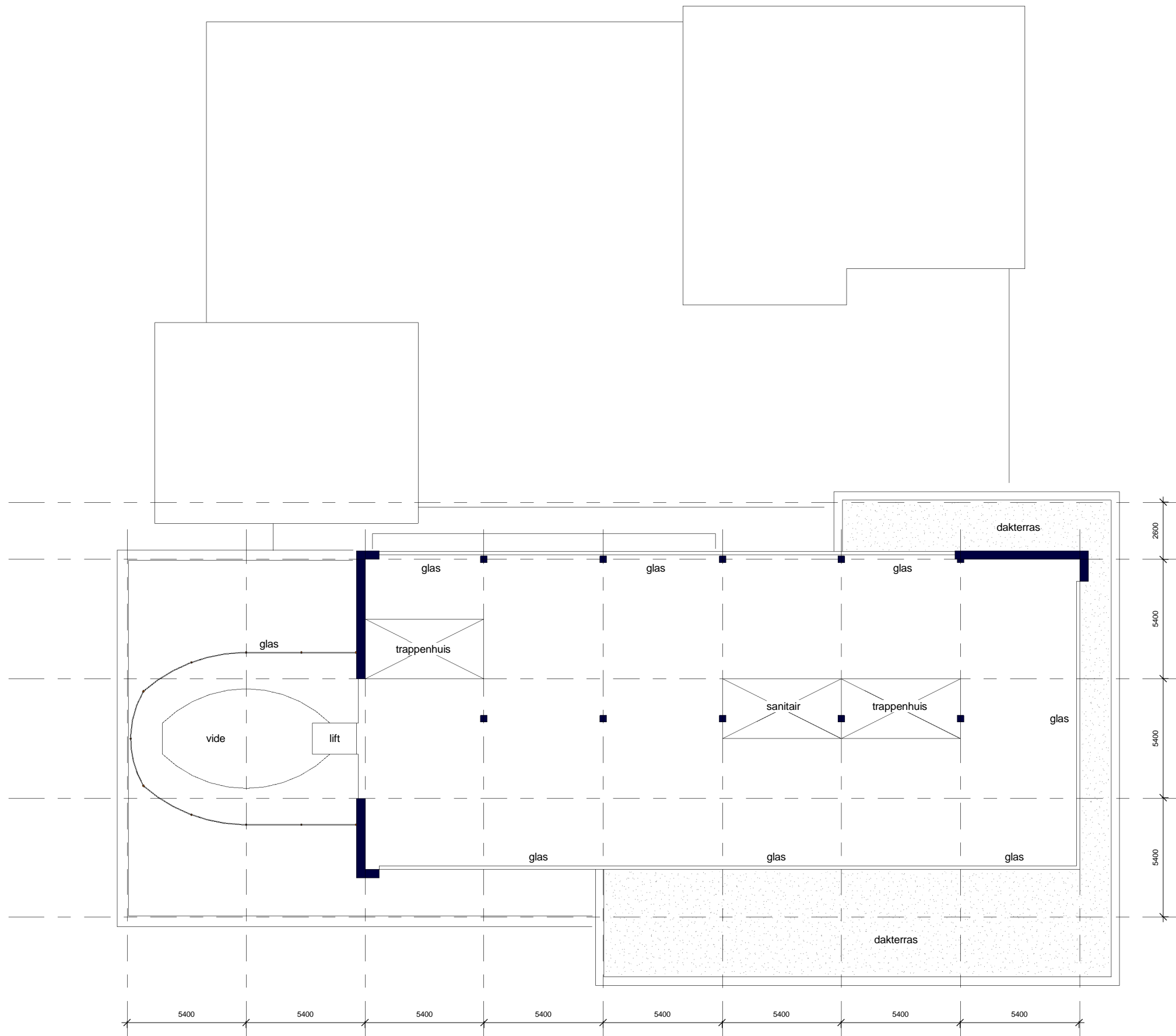
6e VERDIEPING bvo ca. 660 m 2
